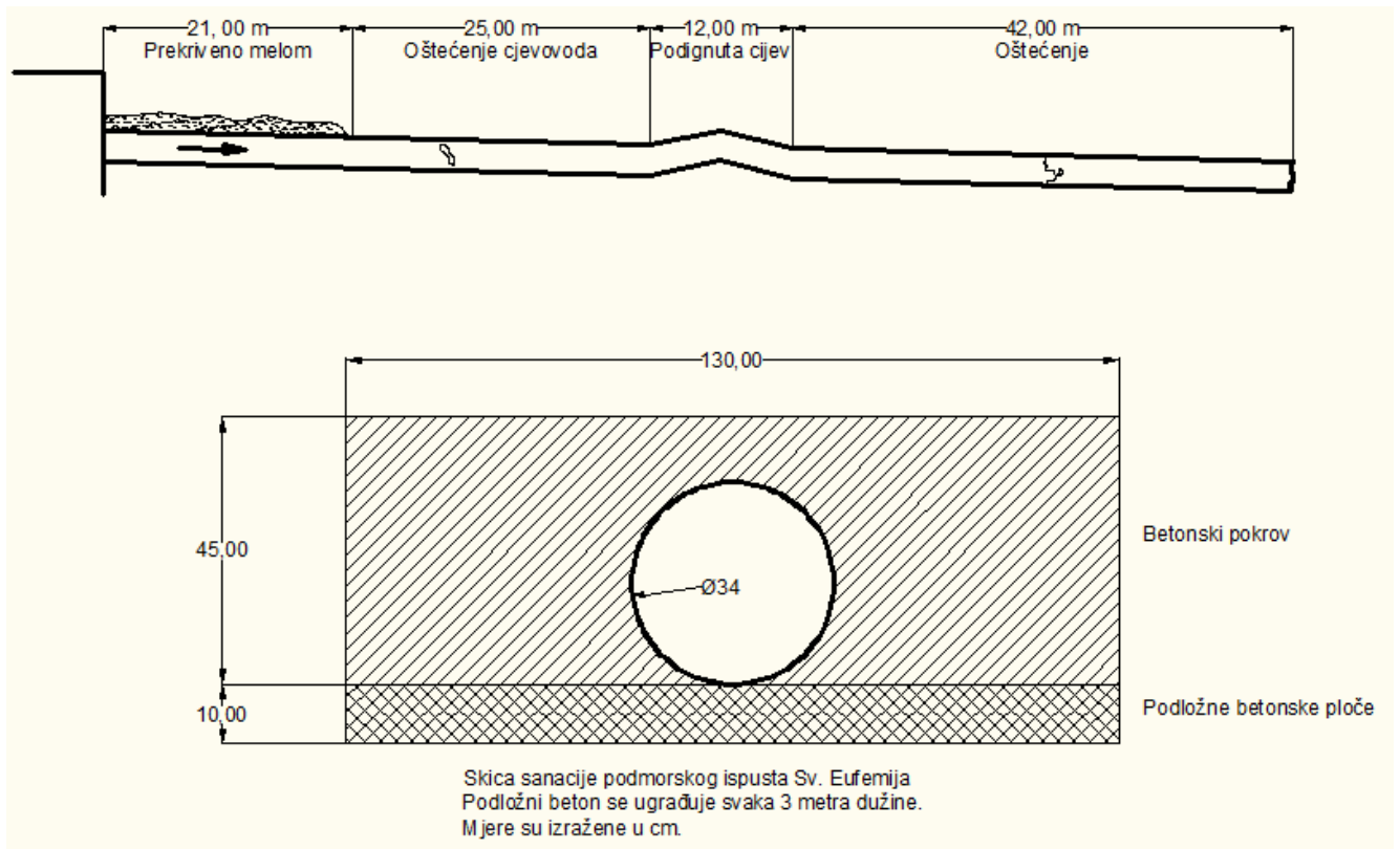
Slika 1 – Skica sanacije podmorskog ispusta Sv. Eufemija
